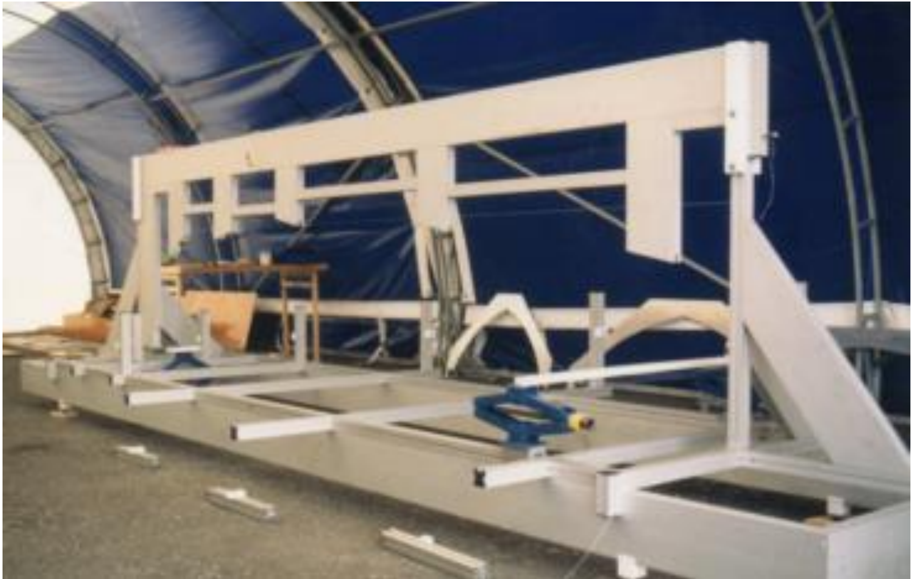
Mätjigg för skrov
